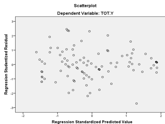
Gambar 1. Uji Heteroskedastisitas
