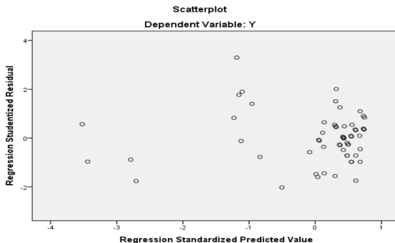
Gambar 1. Uji Heteroskedasitas
