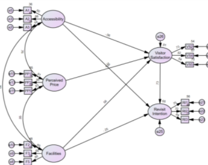
Gambar 4. 3 Uji Hipotesis
