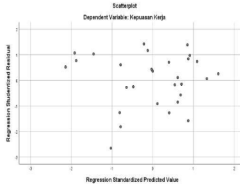
Gambar 2. Grafik Scatterplot
