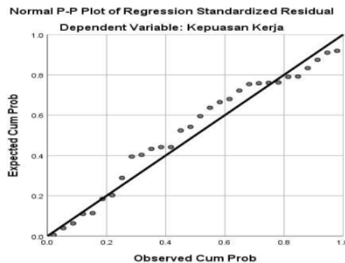
Gambar 1. Grafik Normal PP-Plot
